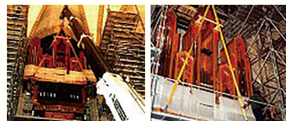
ケース内部のほとんどのパイプや部品を地上で組み立て、中身ごとクレーンで持ちあげた。
